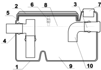
Принципова схема жируловлювача серії СЖ "Оптима"
