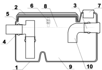
Принципова схема жируюловлювача серії СЖ "Оптима"
